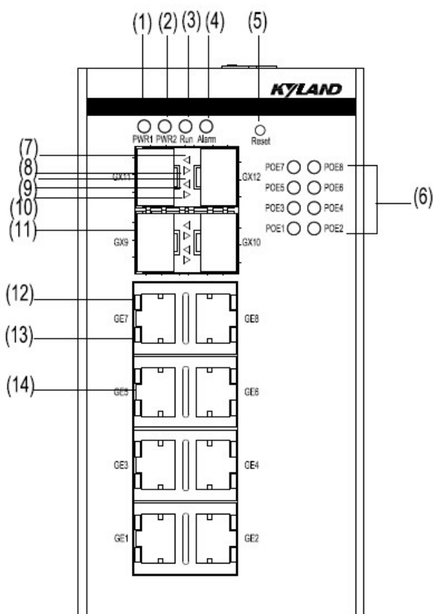
Рисунок 1 Передняя панель
