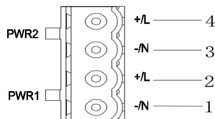
Рисунок 13 4-контактный разъем с расстоянием между контактами 5,08 мм (гнездо)
