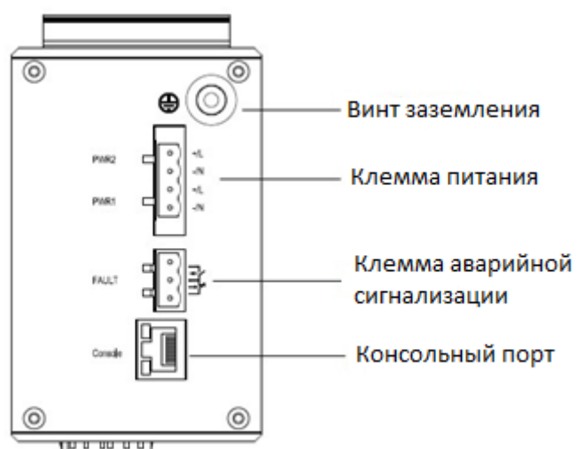
Рисунок 2 Верхняя панель
